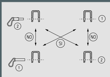
Stützsystem gegen Durchbiegen der Pritsche.
